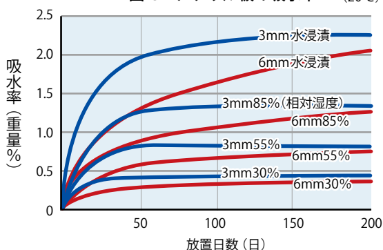
図-3 アクリル板の吸水率 (20℃)
