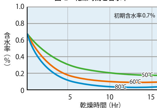
図-2 乾燥時間と含水率
