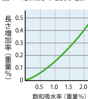
図-5 飽和吸水率と長さ増加率
